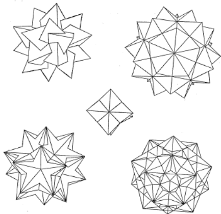
図 6.7 3次元の複合正多面体
